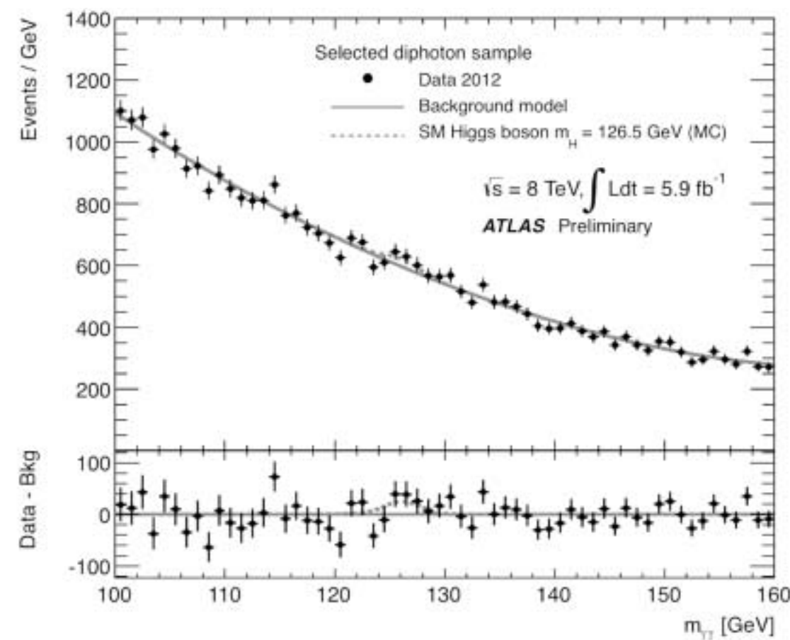
Σχήμα 1: Πειραματικά δεδομένα της ομάδας ATLAS του CERN που «αποδεικνύουν» την ύπαρξη του μποζονίου Χιγκς. Οι μαύρες τελείες-σταυροί είναι οι πειραματικές μετρήσεις με τα σφάλματά τους. Αν ο αναγνώστης συμφωνεί ότι οι μαύρες τελείες προκρίνουν ως πιθανότερη την διακεκομμένη απ' ό,τι την συνεχή καμπύλη, τότε πιστεύει, μαζί με την πλειοψηφία των θεωρητικών φυσικών, ότι ανακαλύφθηκε το μποζόνιο Χιγκς.
